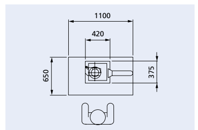
Grundriss SL-2
