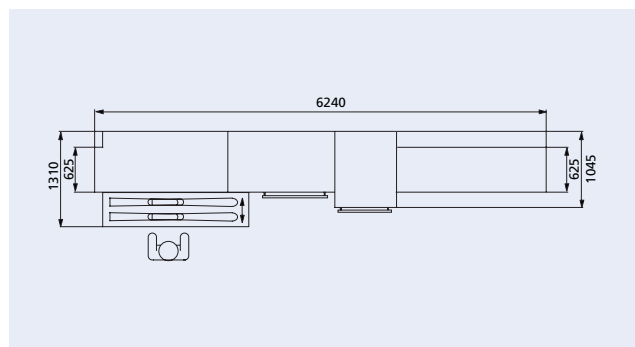
Grundriss SF-2 Pro (ohne automatisches Be- und Entlademagazin)
