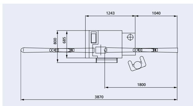
Grundriss PROFI S150
