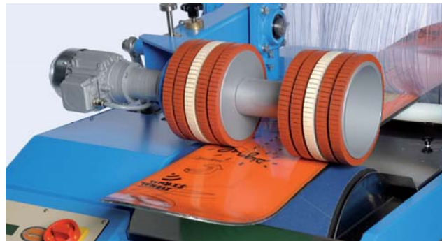
Teilbare Vorschubrolle für perfekte Druckverteilung bei konkaver und konvexer Snowboardsilhouette
