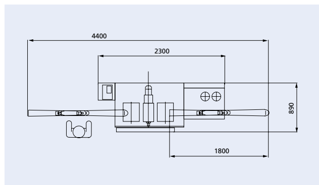
Grundriss PROF I 4
