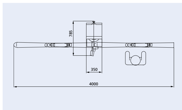
Grundriss KSM-F
